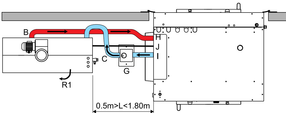
Plassering av gassutveksleren på høyre side av vaske- og sentrifugeringsmaskinen Du kan rotere den 90 ° (R1)
